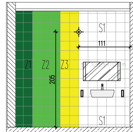
WIDOK S7
