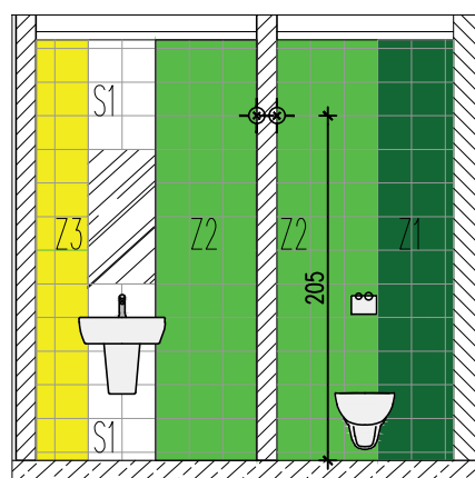
WIDOK S6
