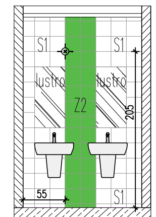
WIDOK S3
