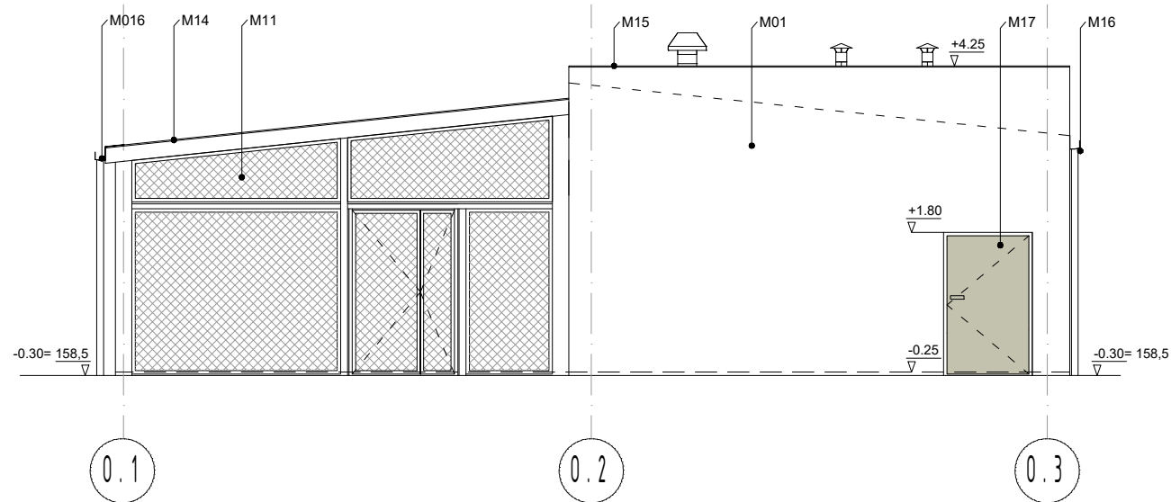
ELEWACJA ZACHODNIA
