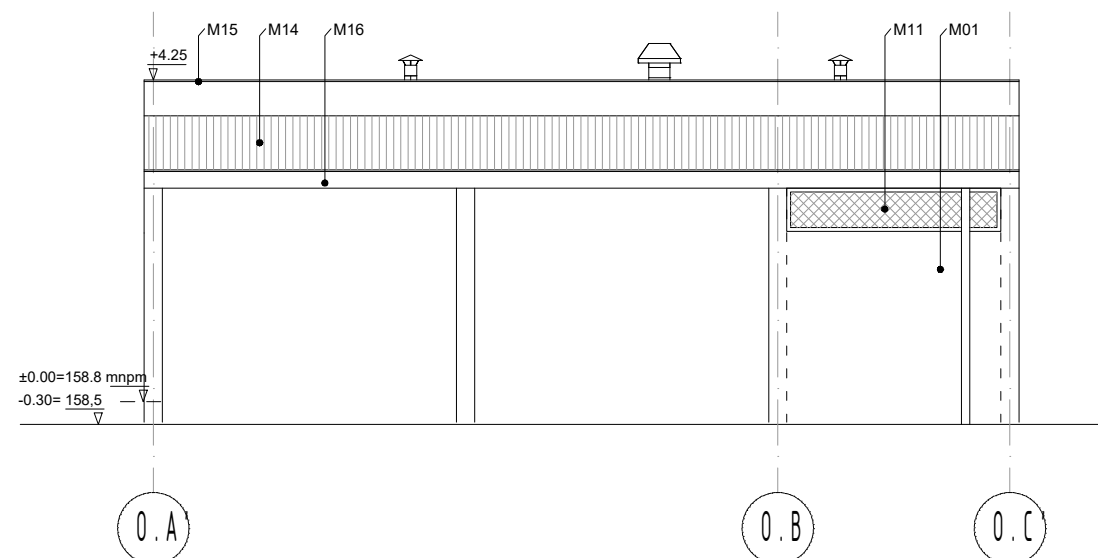
ELEWACJA PÓŁNOCNO-ZACHODNIA
