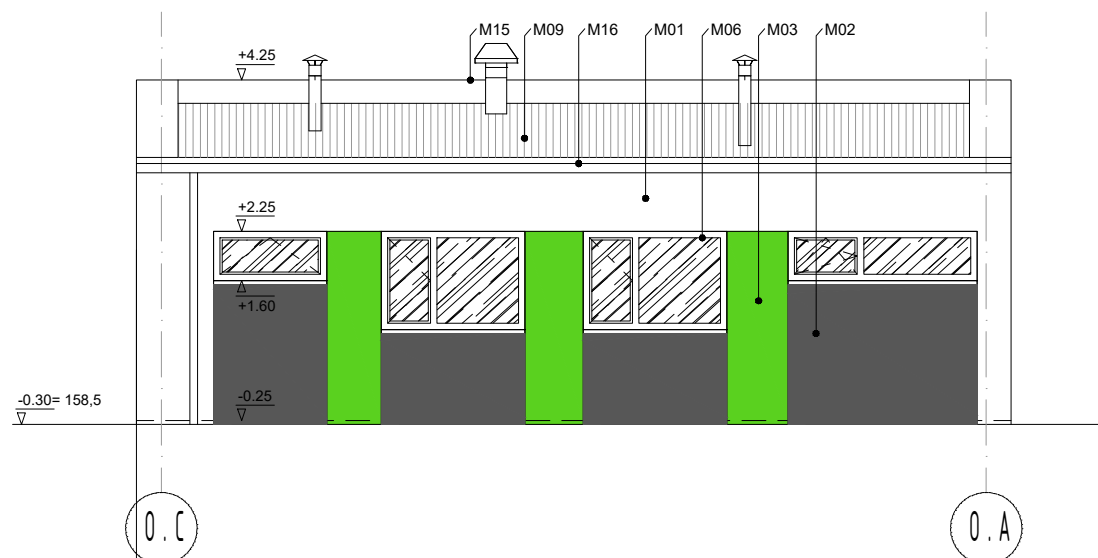
ELEWACJA POŁUDNIOWO-WSCHODNIA
