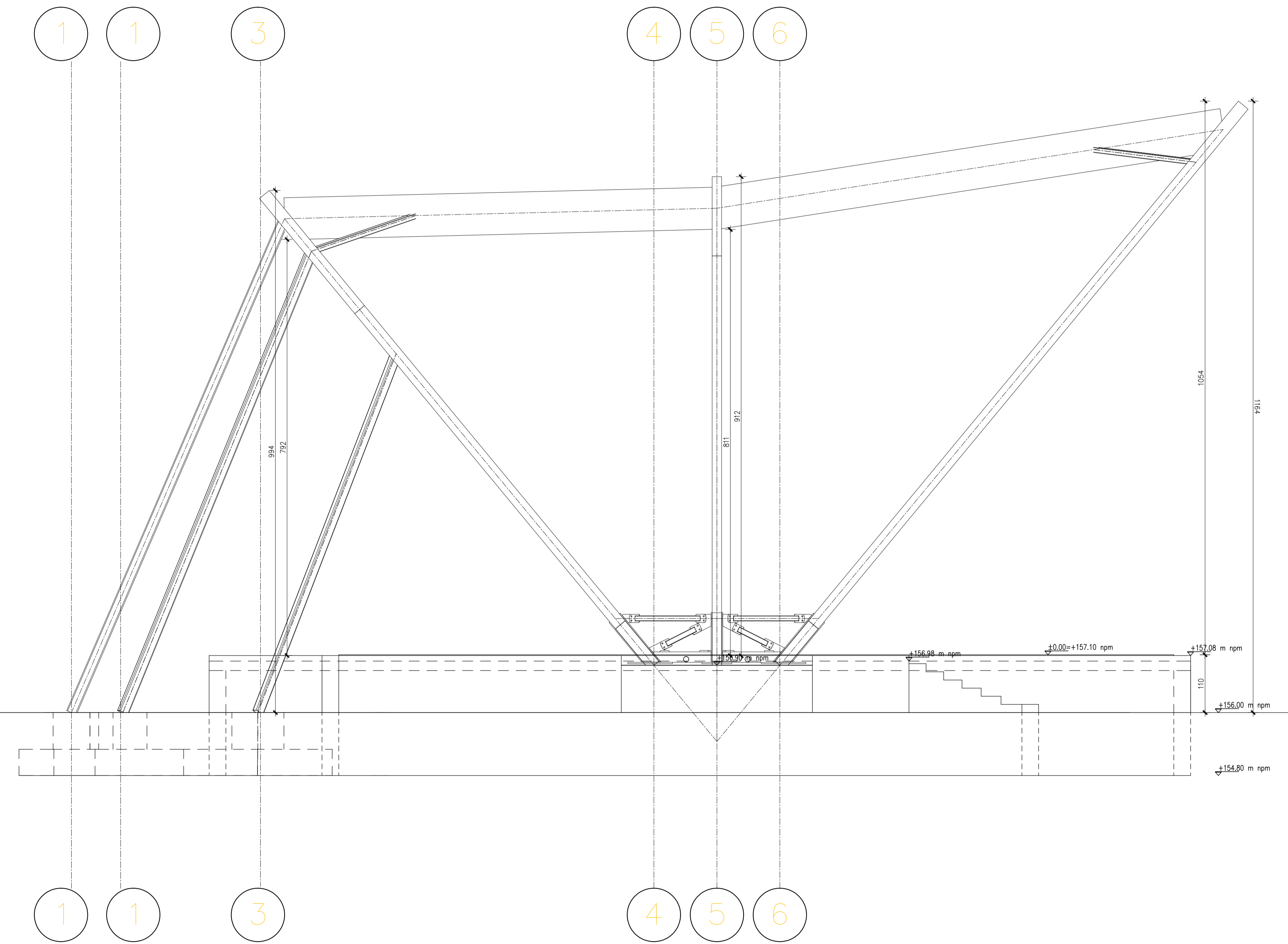
PRZEKRÓJ A-A
