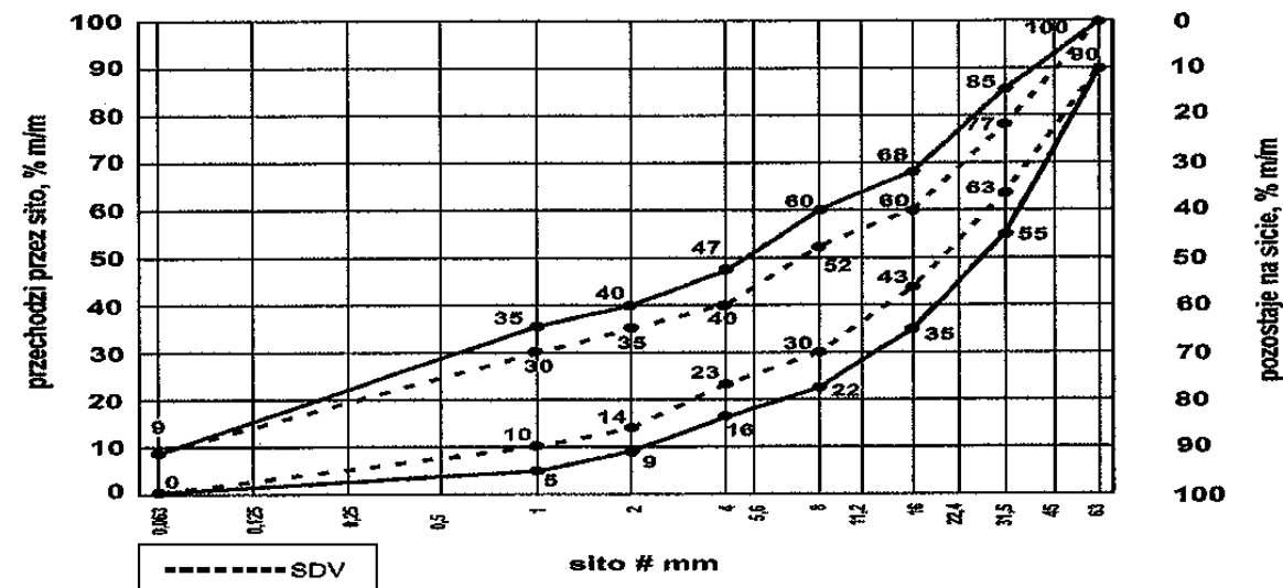
Rys. 2. Krzywe graniczne uziarnienia mieszanki kruszywa niezwiązanego 0/63 mm do warstwy podbudowy zasadniczej
