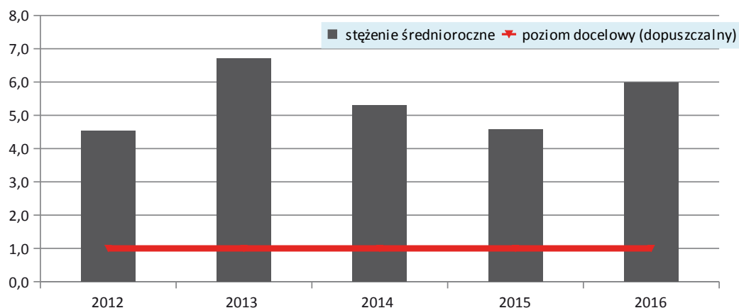
Rys. 3.3 Stężenie średnioroczne benzo(a)pirenu na stacji pomiarowej w Łodzi przy ul. Legionów 1 w latach 2012–2016
