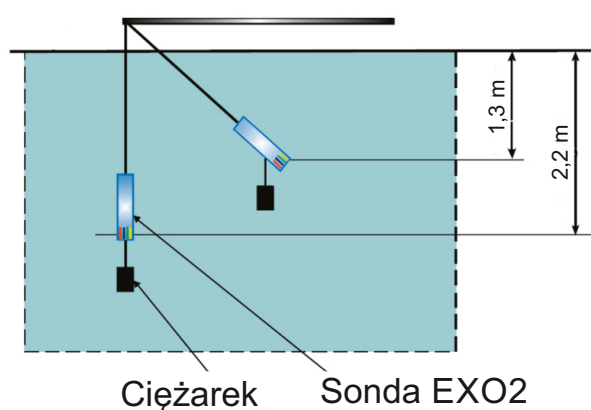
Rys. 2.13 Schemat montażu i fotografia mobilnego systemu pomiarów monitoringowych.
