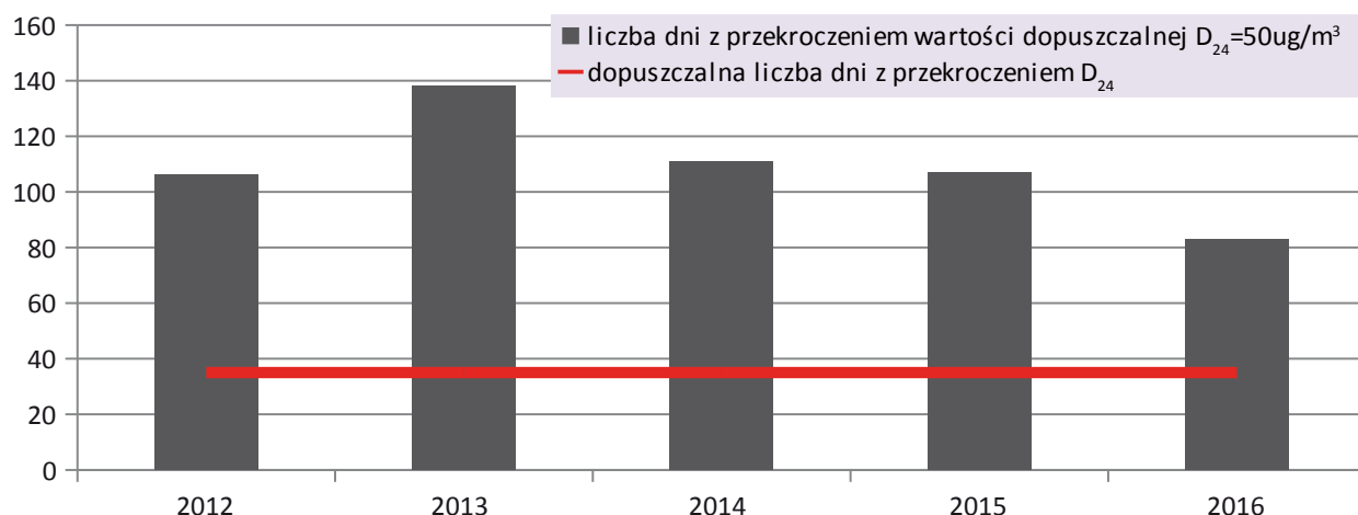
Rys. 3.2 Liczba dni z przekroczeniem wartości dopuszczalnej średniodobowej D_{24} pyłu PM_{10} na stacji pomiarowej w Łodzi przy ul. Legionów 1 w latach 2012–2016
